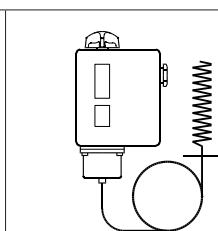
Fig. 2 Thermostat à bulbe de gaine
